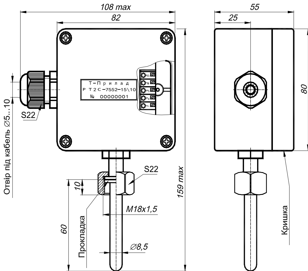
Малюнок 1 – Габаритні розміри РТ2С-7552.
