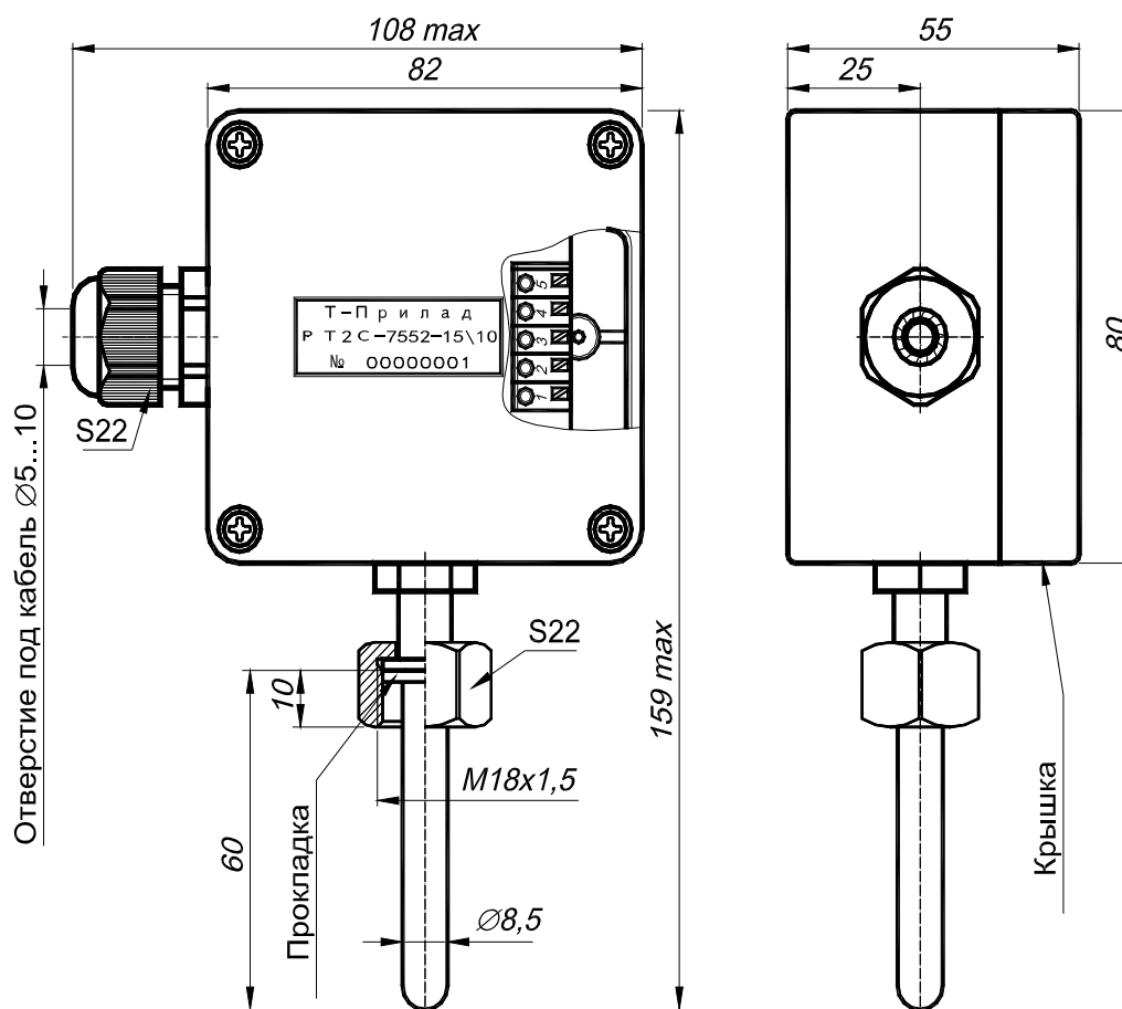
Рисунок 1 – Габаритные размеры PT2C-7552.
