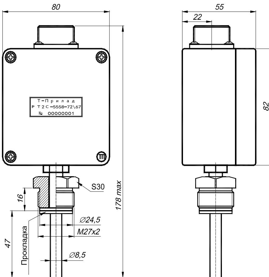
Малюнок 1 – Габаритні розміри РТ2С-5558.
