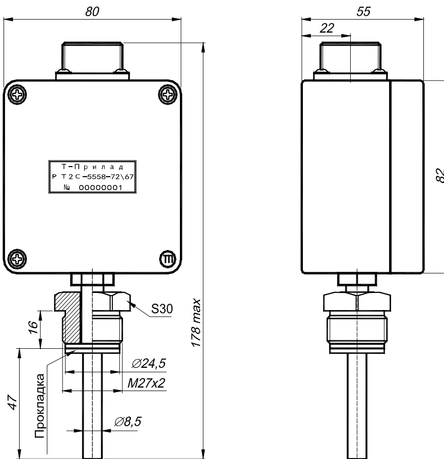
Рисунок 1 – Габаритные размеры PT2C-5558.
