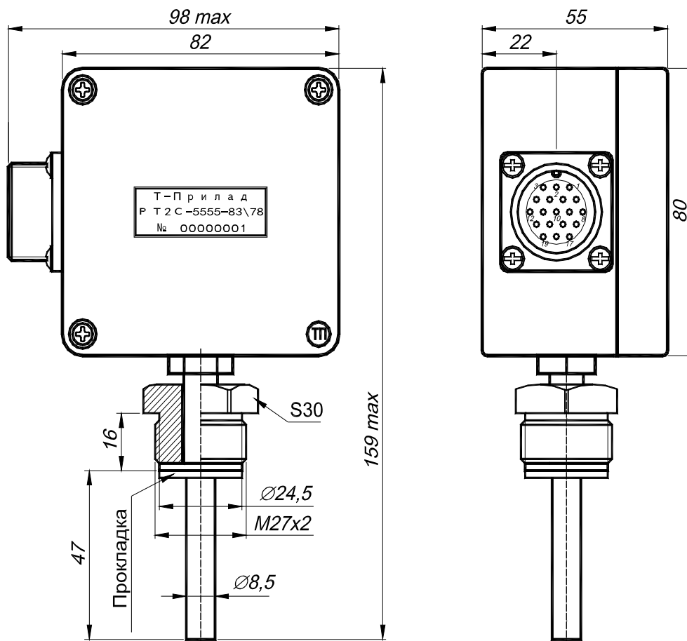
Малюнок 1 – Габаритні розміри РТ2С-5555.
