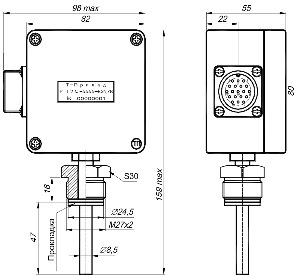
Рисунок 1 – Габаритные размеры PT2C-5555.
