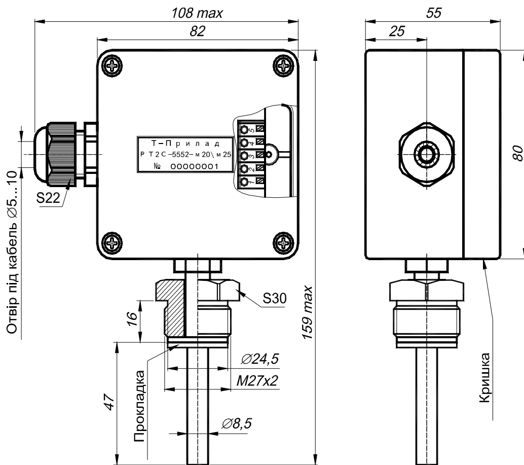
Малюнок 1 – Габаритні розміри РТ2С-5552.
