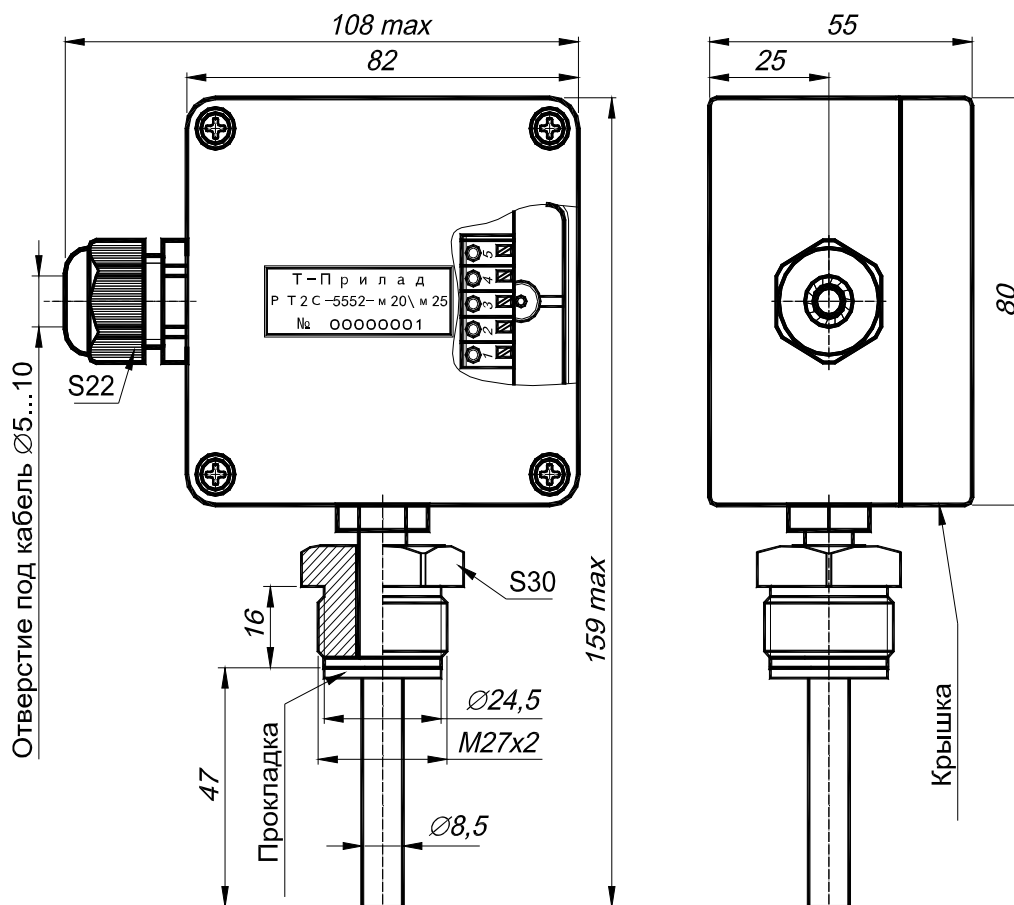
Рисунок 1 – Габаритные размеры PT2C-5552.
