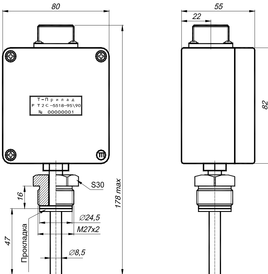
Малюнок 1 – Габаритні розміри PT2C-5518.
