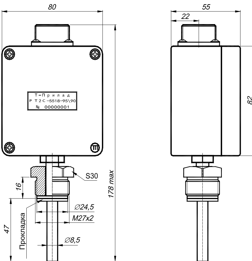
Рисунок 1 – Габаритные размеры PT2C-5518.
