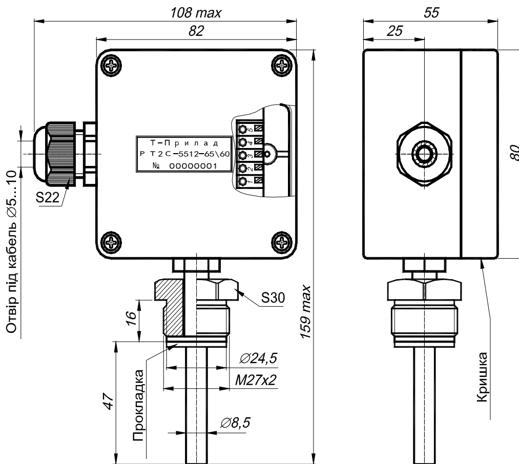
Малюнок 1 – Габаритні розміри РТ2С-5512.
