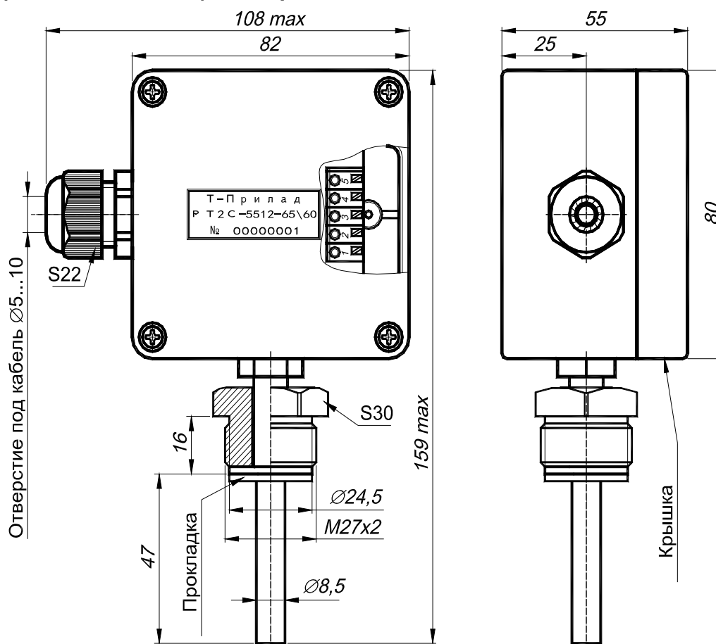
Рисунок 1 – Габаритные размеры PT2C-5512.
