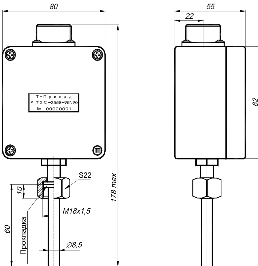
Малюнок 1 – Габаритні розміри РТ2С-2558.
