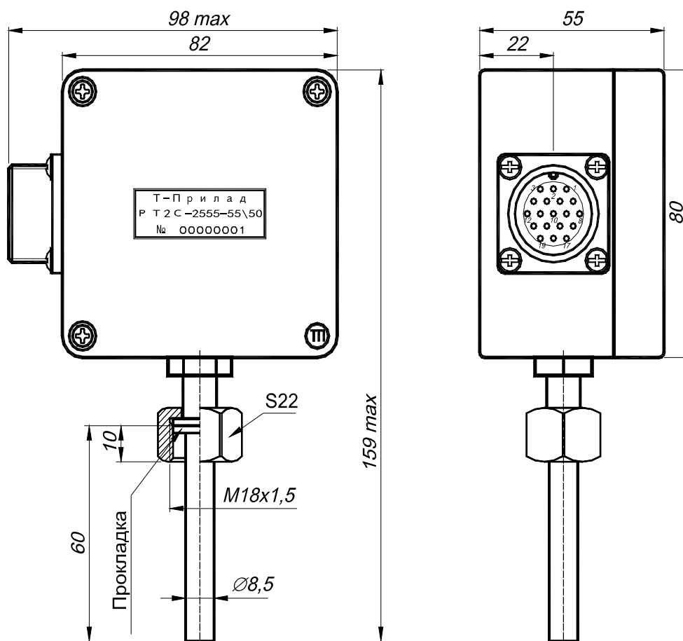
Рисунок 1 – Габаритные размеры РТ2С-2555.
