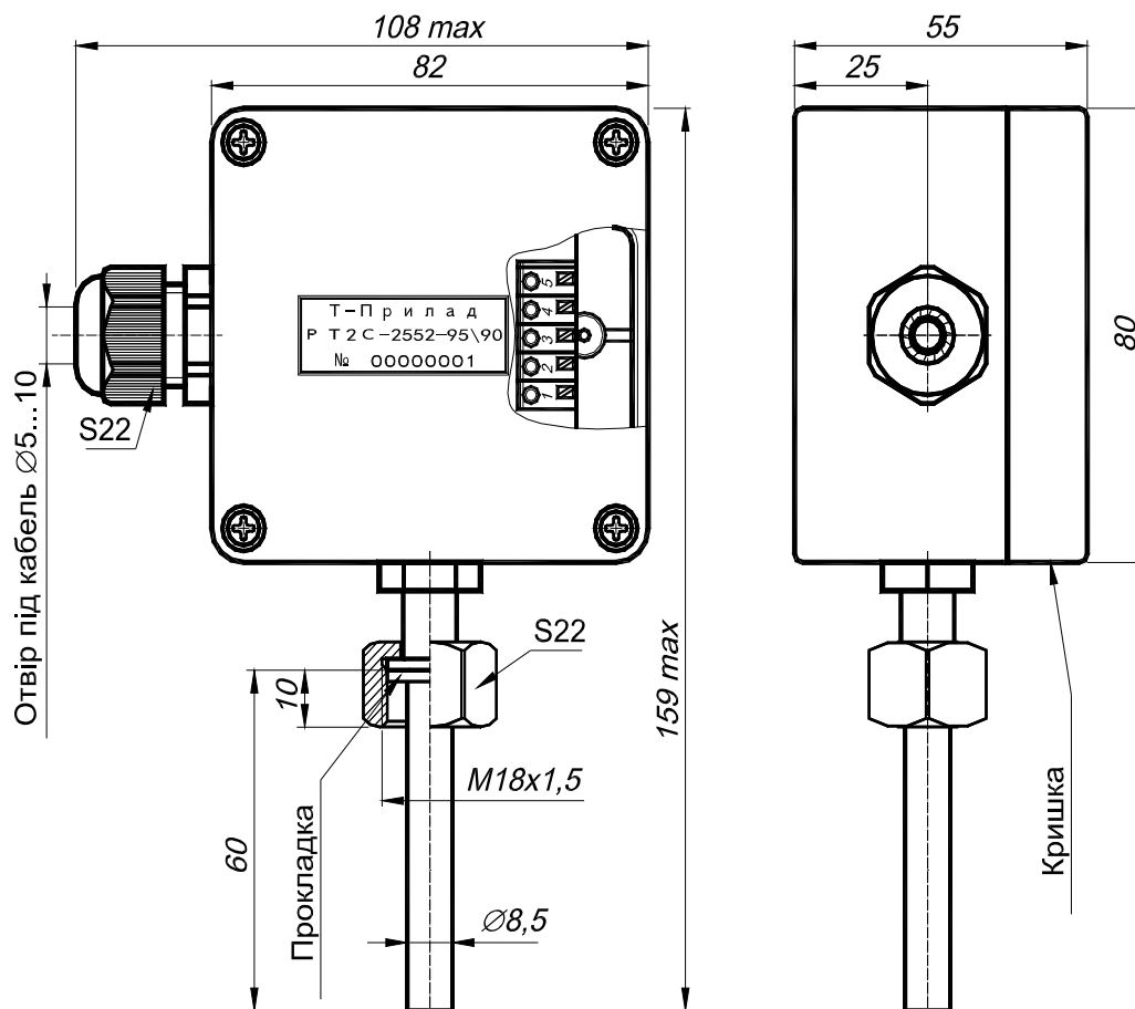
Малюнок 1 – Габаритні розміри РТ2С-2552.
