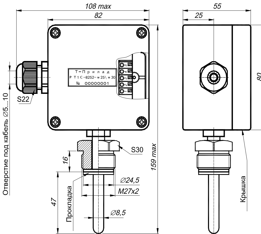
Рисунок 1 – Габаритные размеры PT1C-8252.
