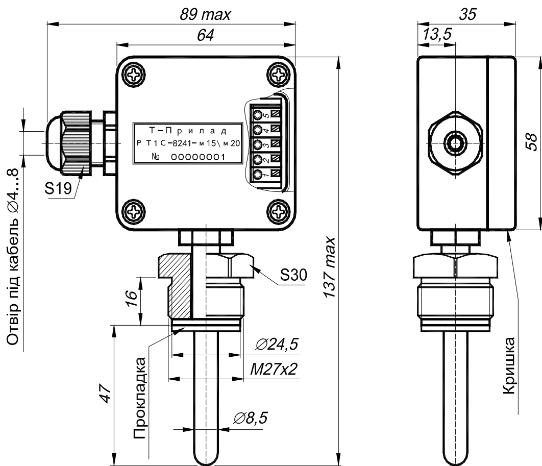
Малюнок 1 – Габаритні розміри РТ1С-8241.
