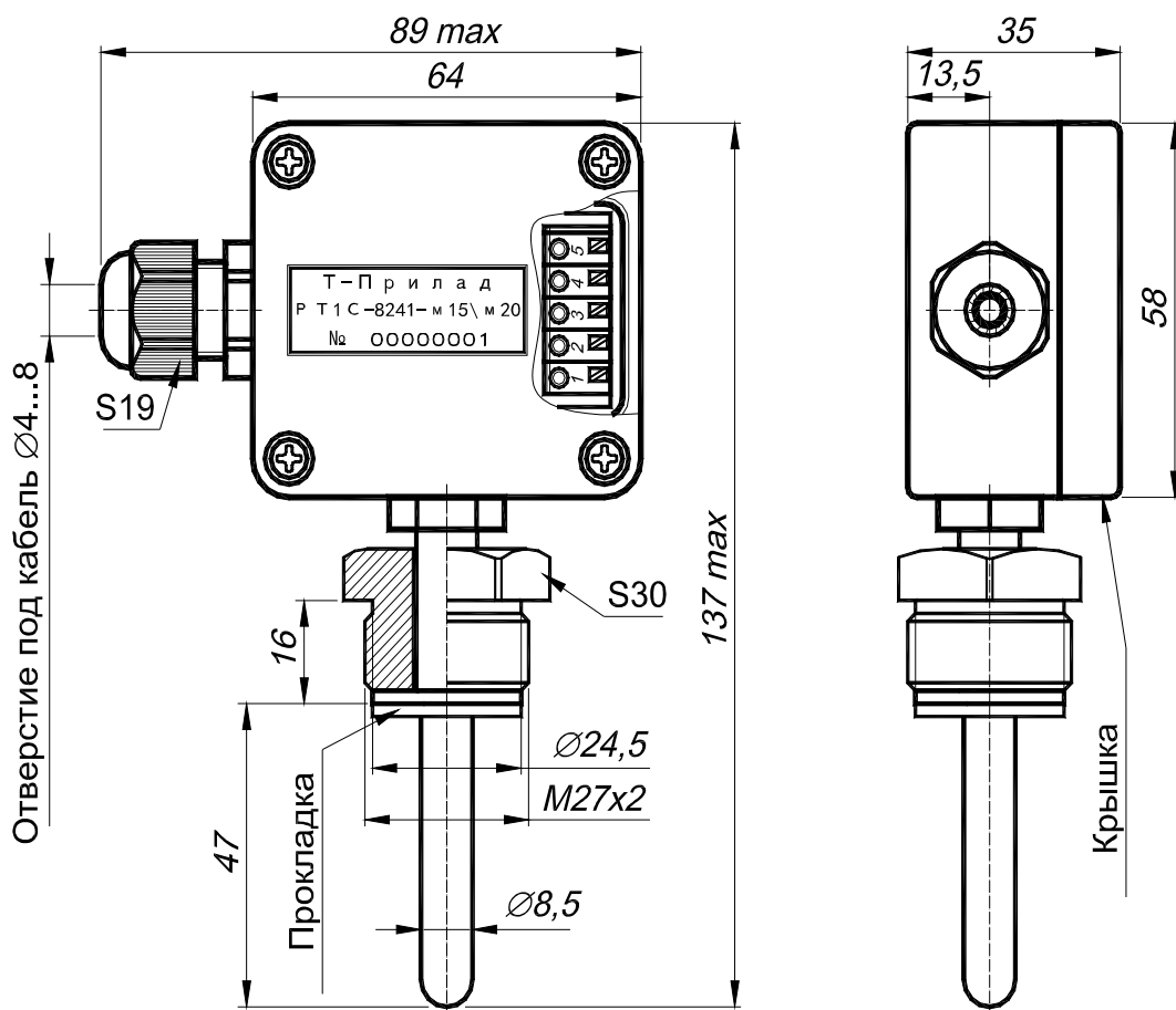
Рисунок 1 – Габаритные размеры РТ1С-8241.
