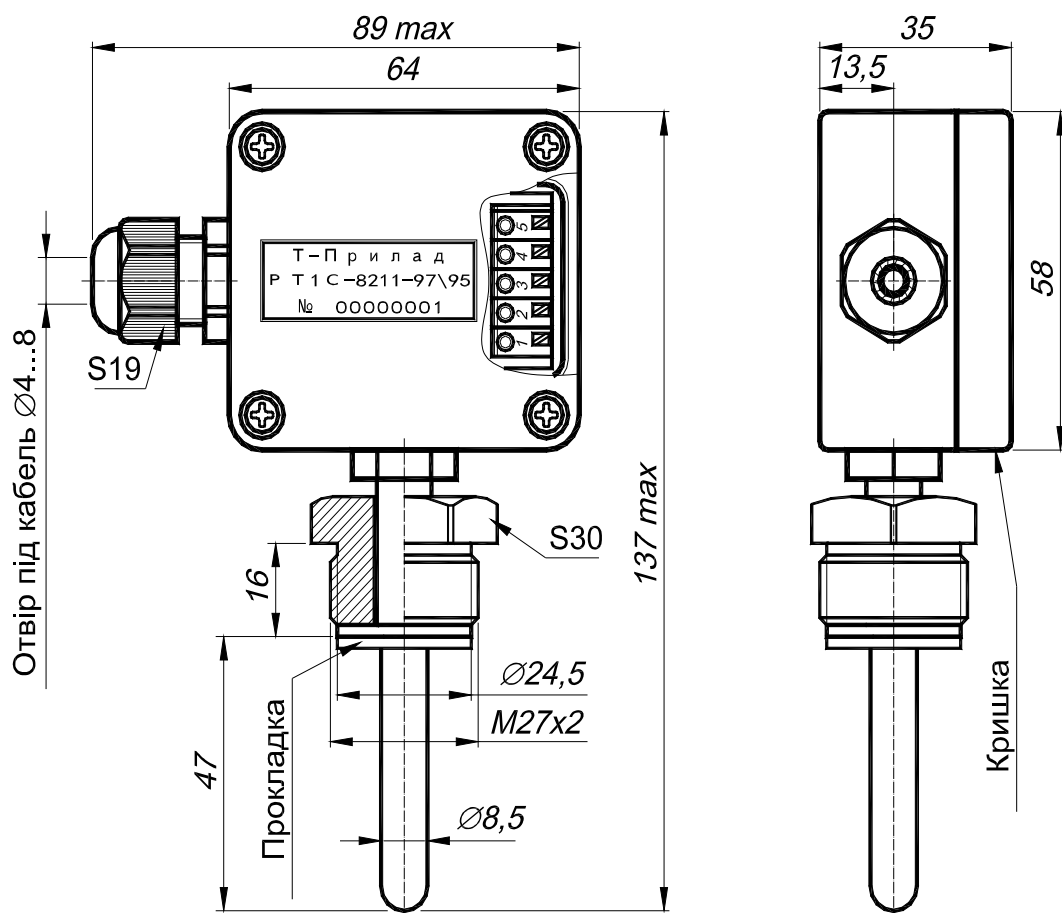
Малюнок 1 – Габаритні розміри РТ1С-8211.
