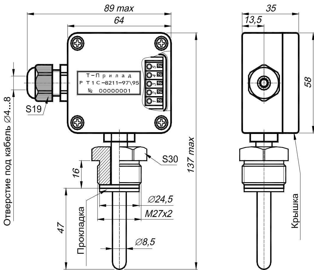
Рисунок 1 – Габаритные размеры PT1C-8211.
