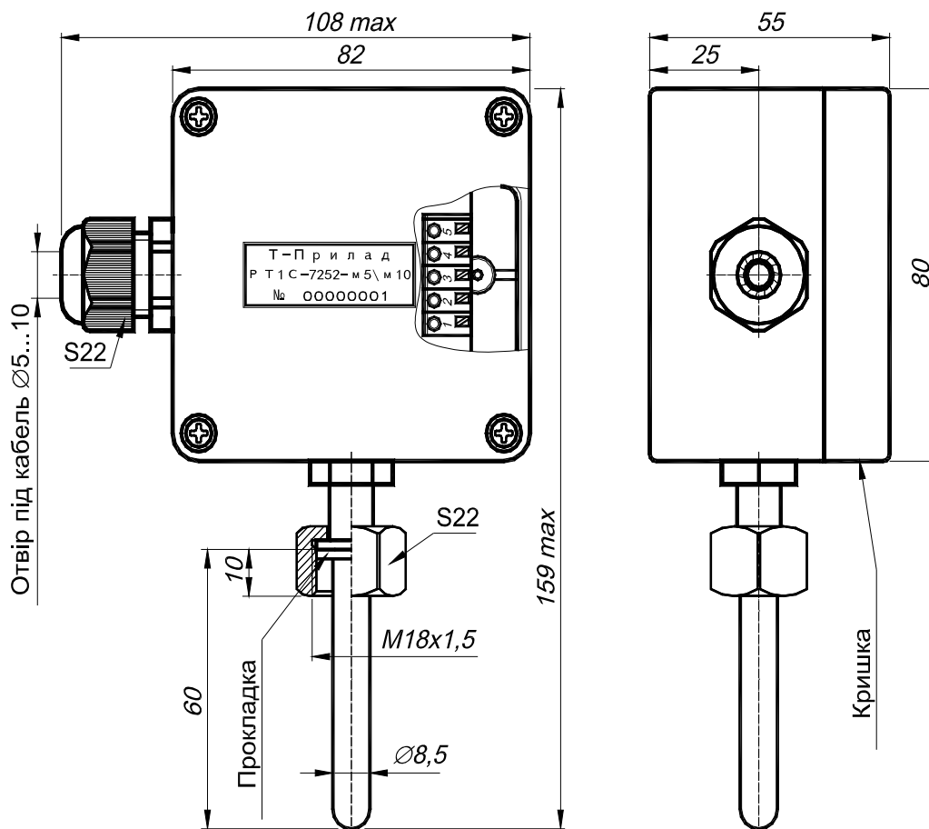
Малюнок 1 – Габаритні розміри РТ1С-7252.
