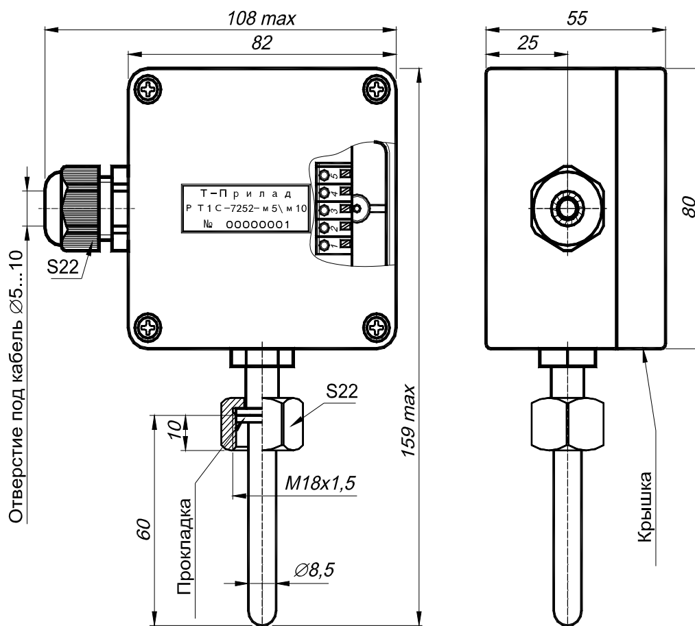
Рисунок 1 – Габаритные размеры PT1C-7252.
