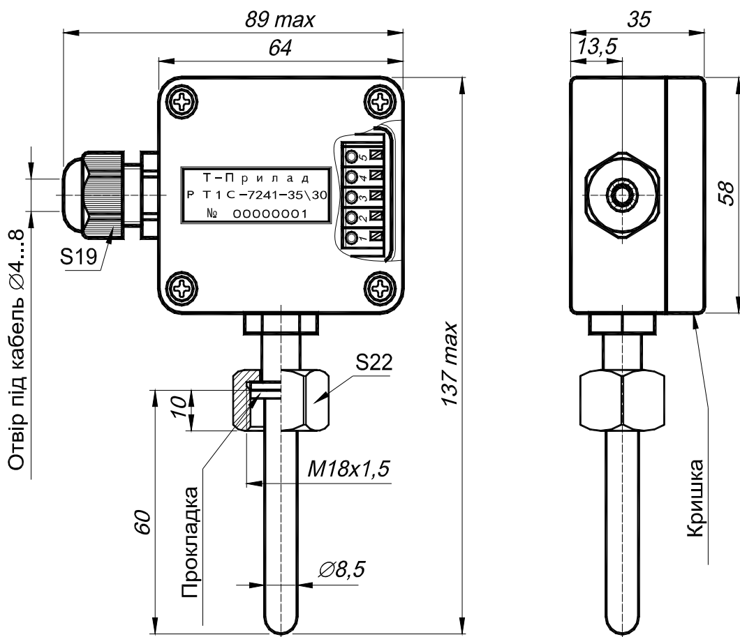
Малюнок 1 – Габаритні розміри РТ1С-7241.
