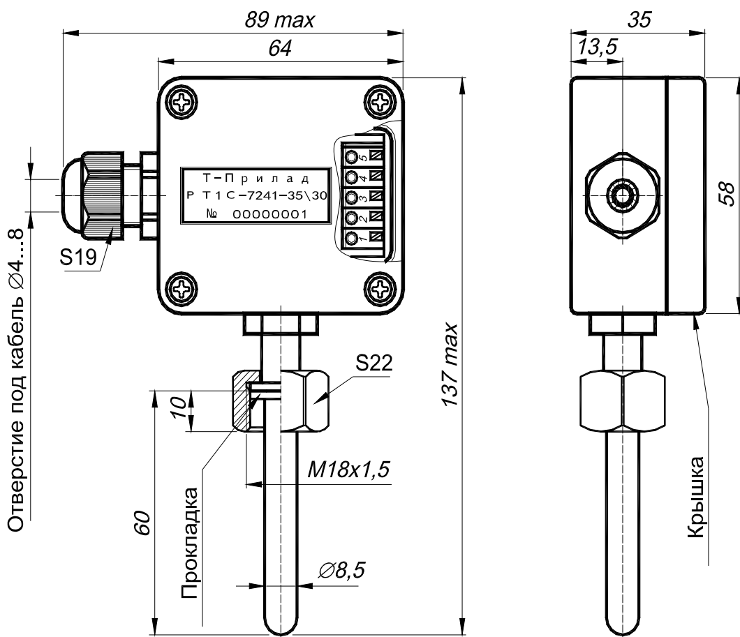
Рисунок 1 – Габаритные размеры РТ1С-7241.
