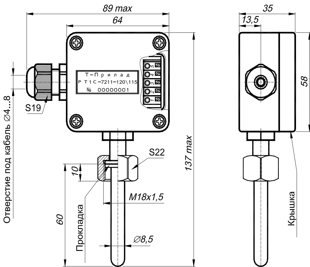
Рисунок 1 – Габаритные размеры РТ1С-7211.
