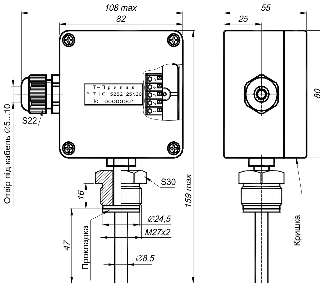
Малюнок 1 – Габаритні розміри РТ1С-5252.
