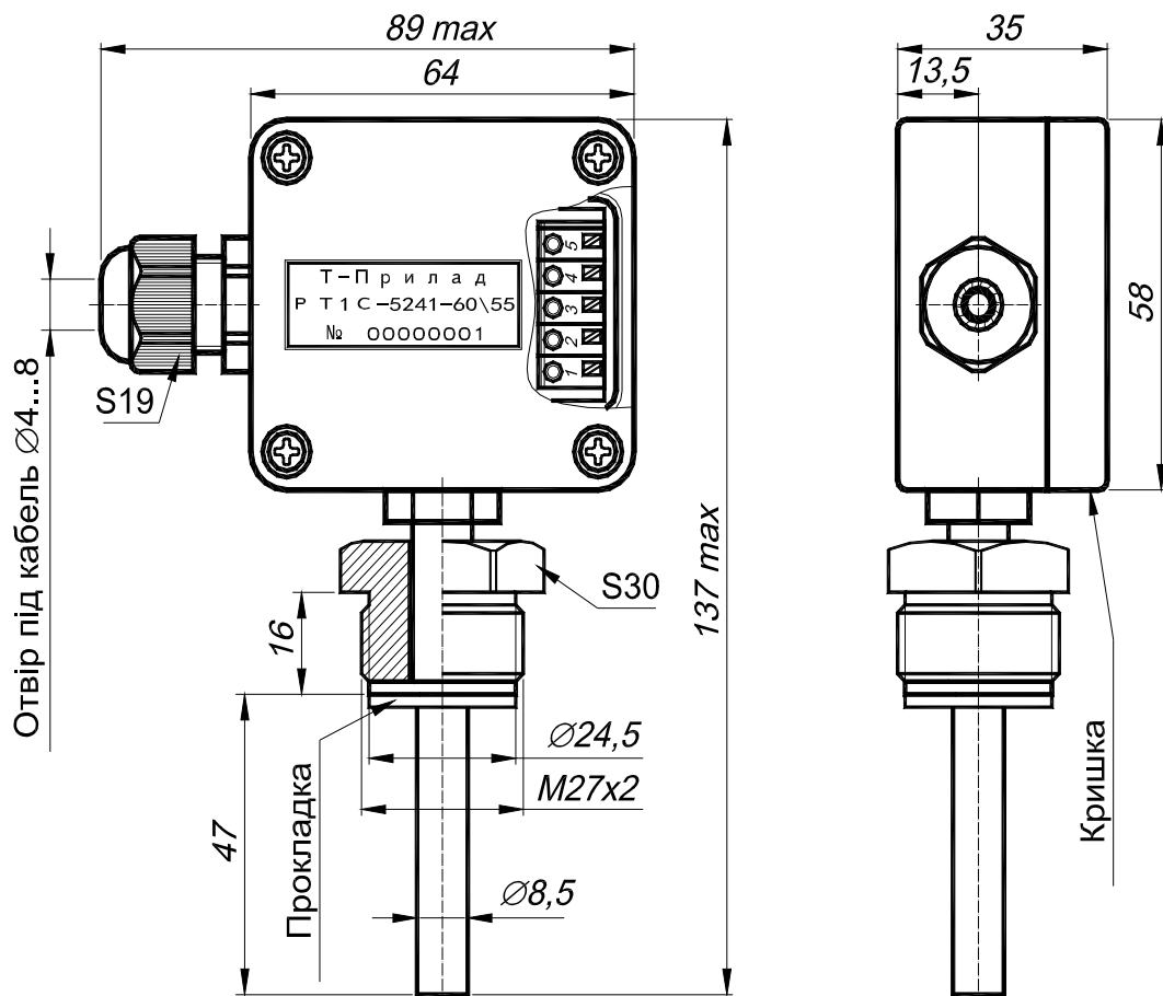
Малюнок 1 – Габаритні розміри РТ1С-5241.
