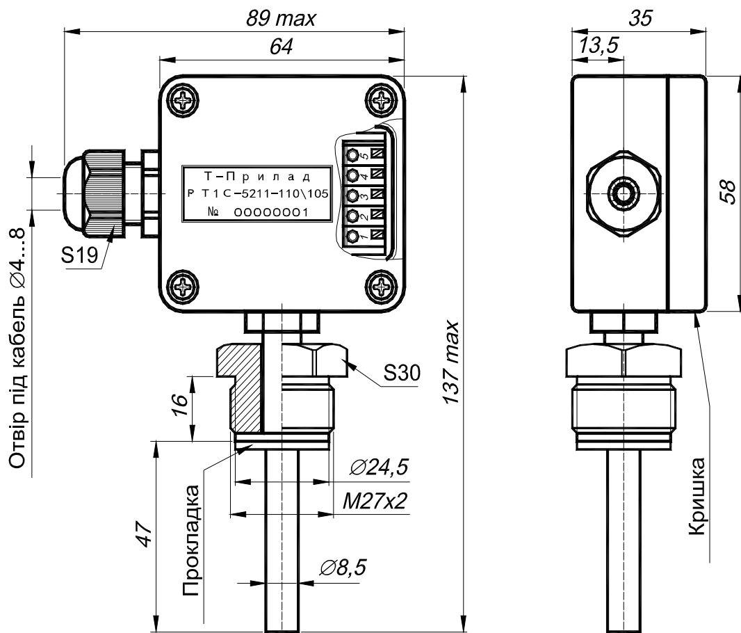
Малюнок 1 – Габаритні розміри РТ1С-5211.
