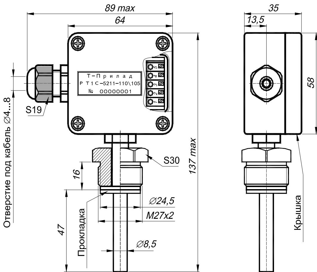
Рисунок 1 – Габаритные размеры РТ1С-5211.
