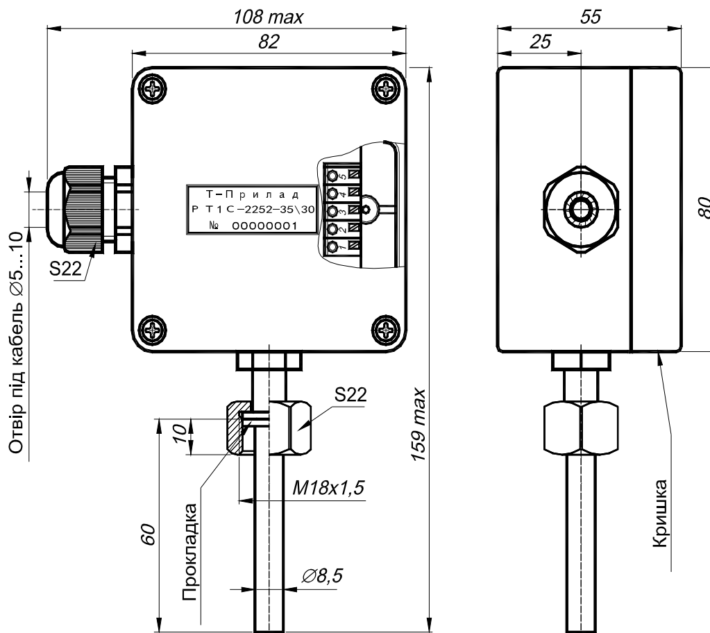
Малюнок 1 – Габаритні розміри РТ1С-2252.
