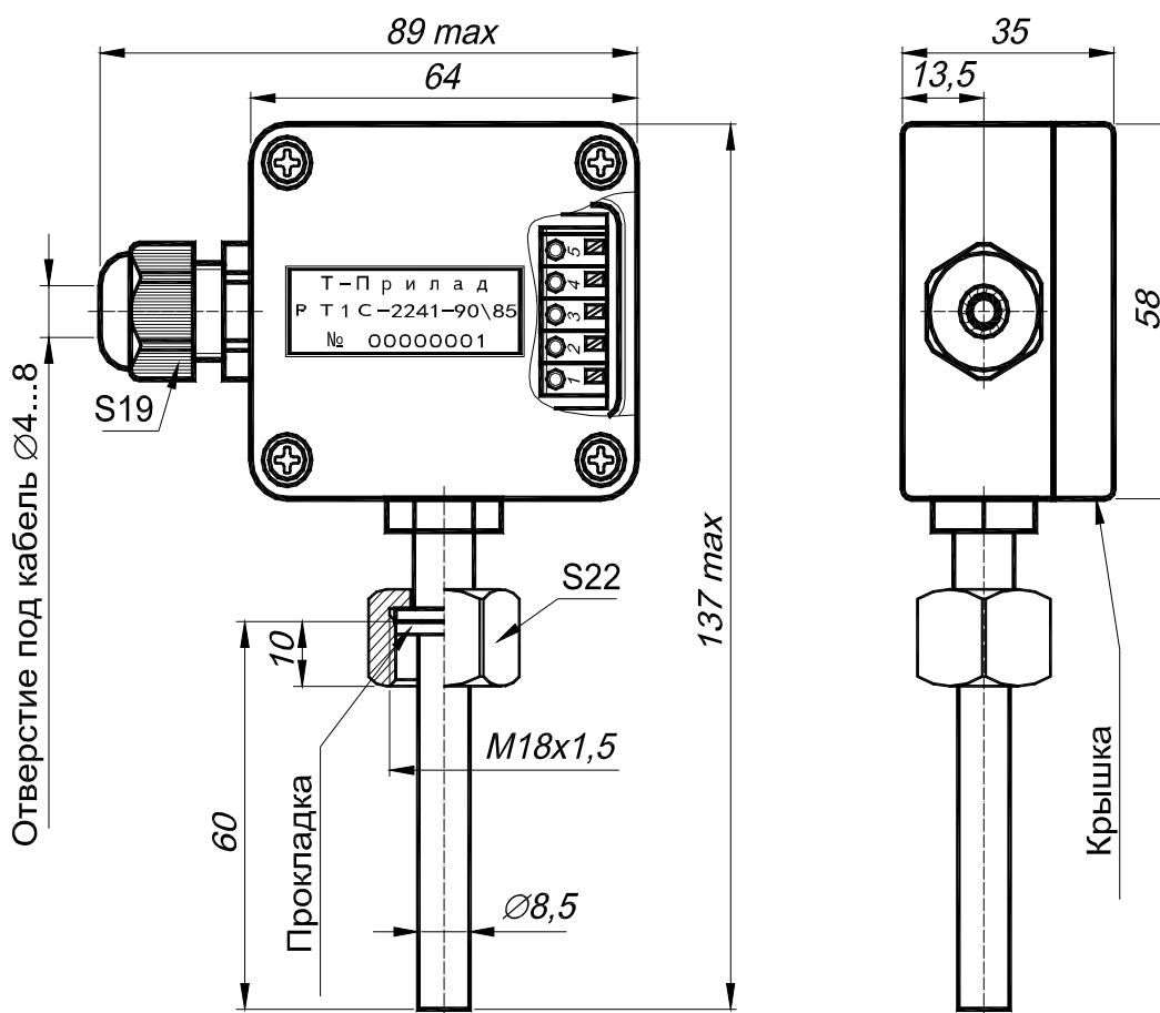
Рисунок 1 – Габаритные размеры РТ1С-2241.
