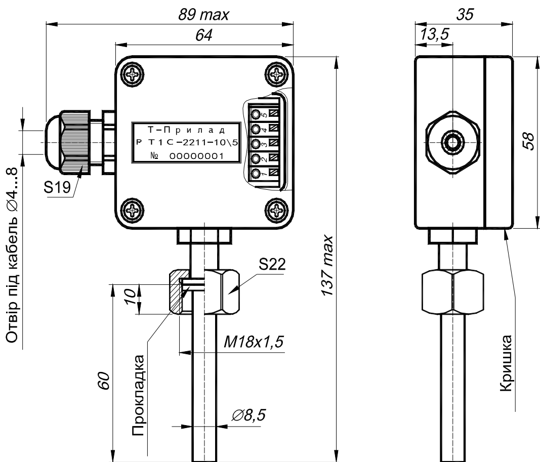
Малюнок 1 – Габаритні розміри РТ1С-2211.
