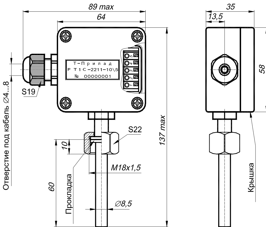
Рисунок 1 – Габаритные размеры РТ1С-2211.
