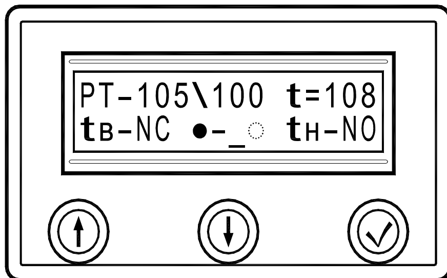
Малюнок 1 – Ескіз лицьової панелі ПРТ1С у режимі контролю.
