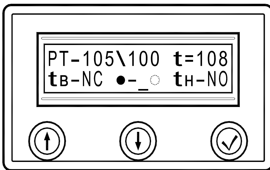
Рисунок 1 – Эскиз лицевой панели ПРТ1С в режиме контроля.
